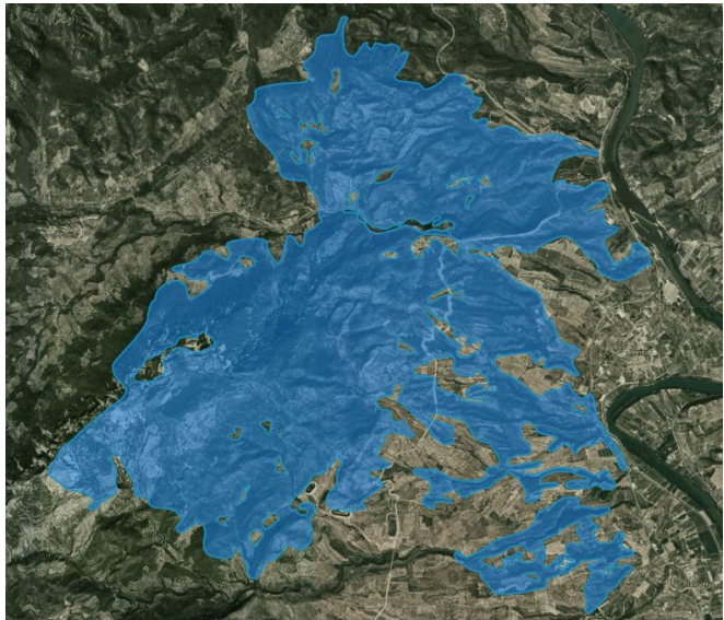
IIF en Paüls (Tarragona) [Cataluña] 07/07/2025 Imagen por satélite del área afectada Fuente: Effis - Copernicus
